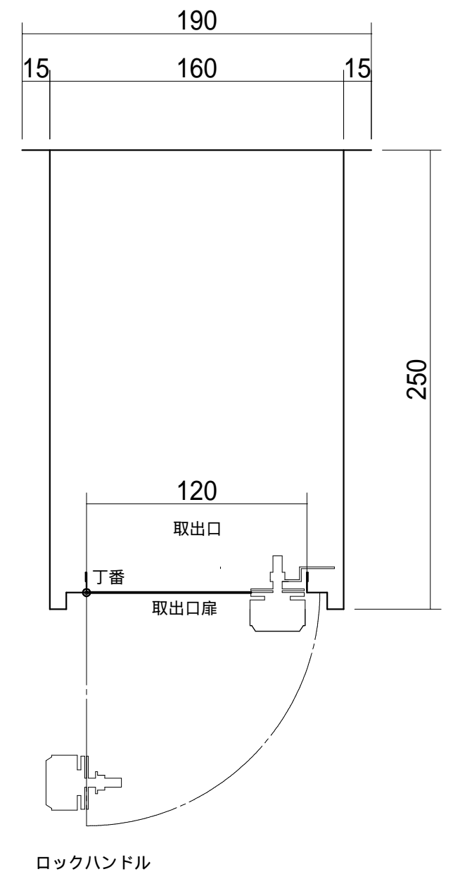
上面断面図
